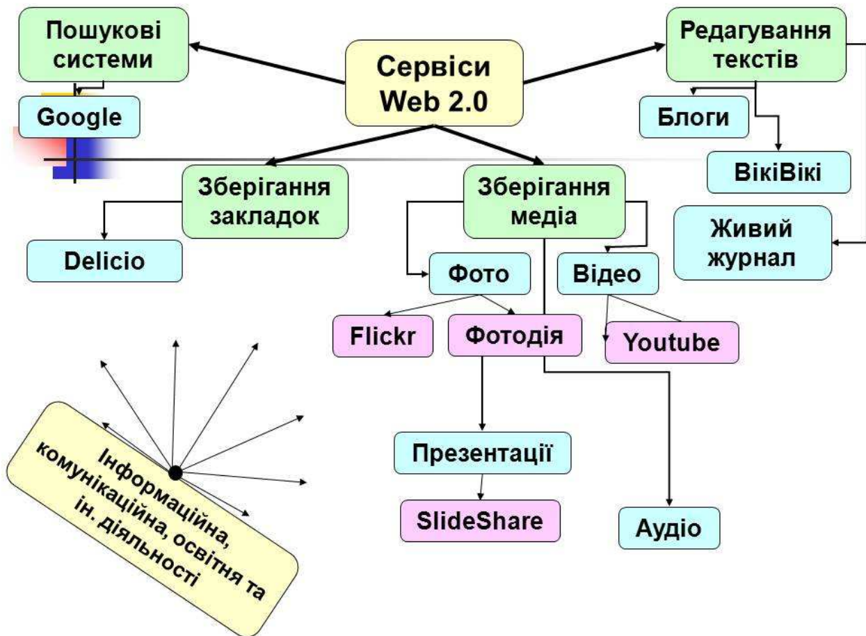
Рис. 1. Сервіси Web 2.0
